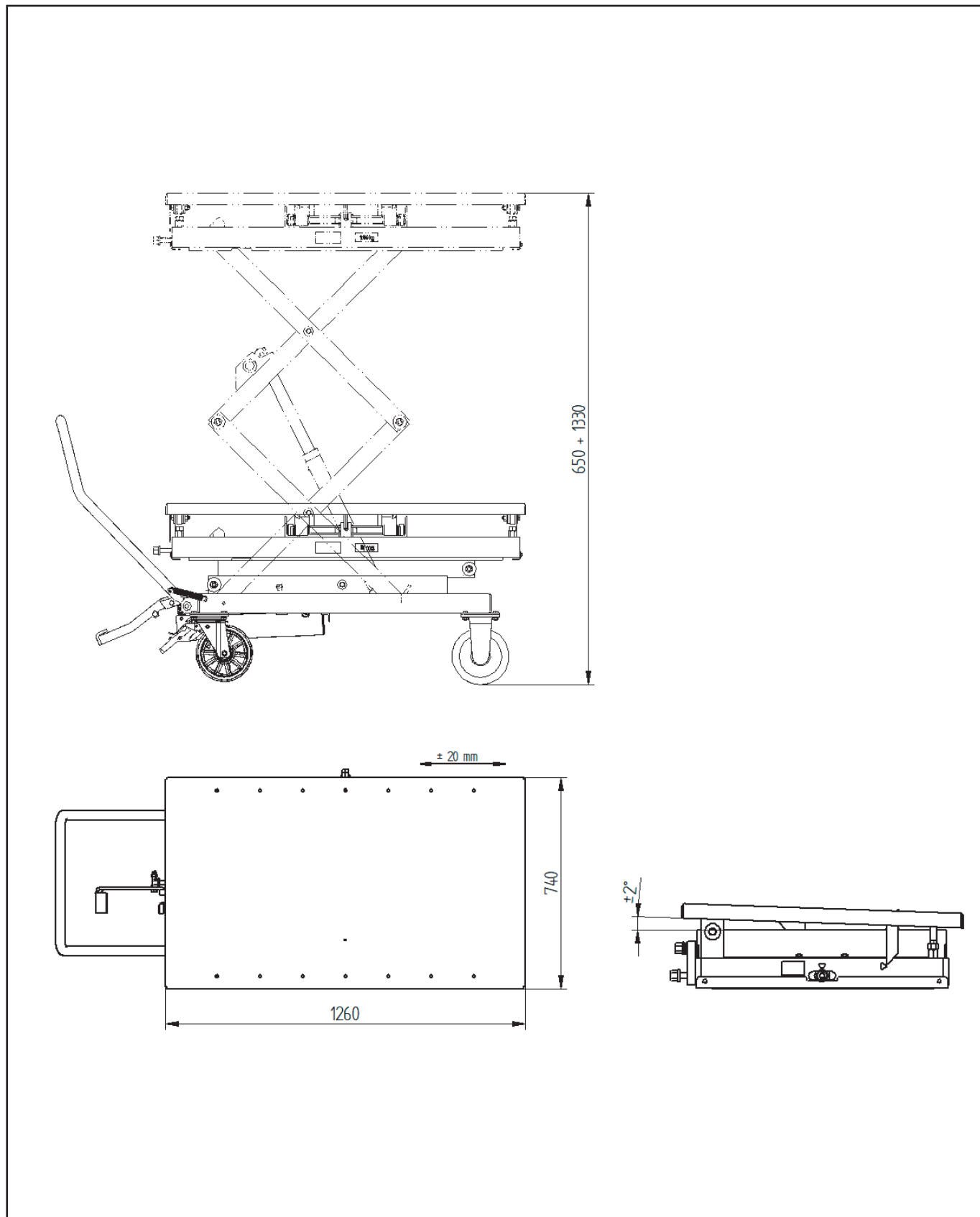
Габаритный чертеж Master Gear 1.0
