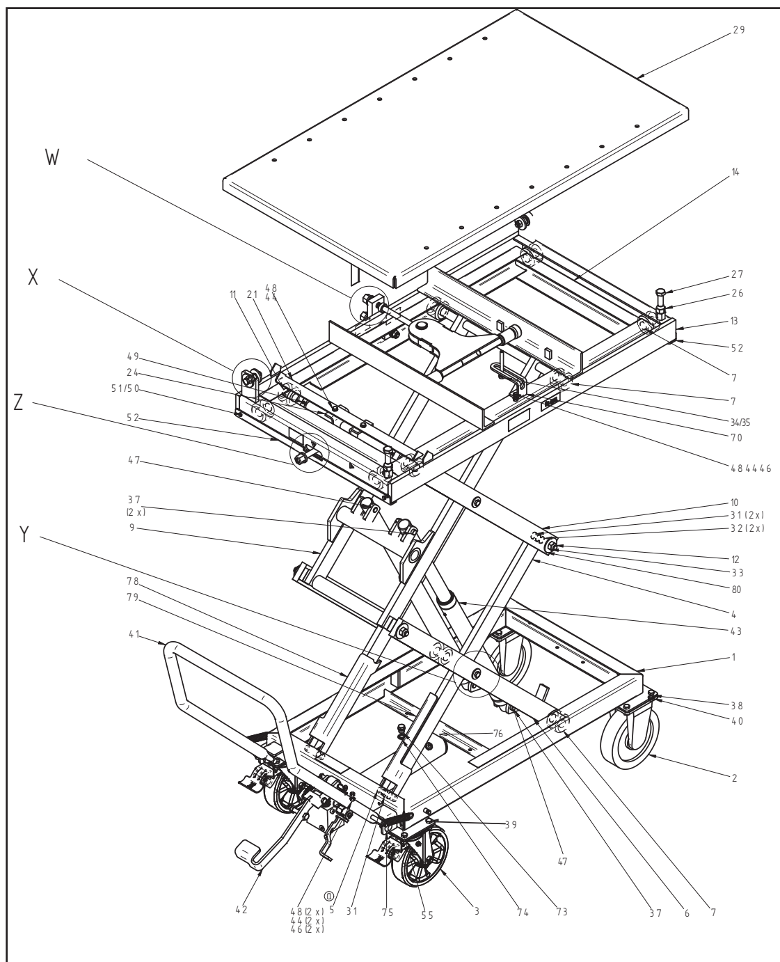
Габаритный чертеж 1.0
