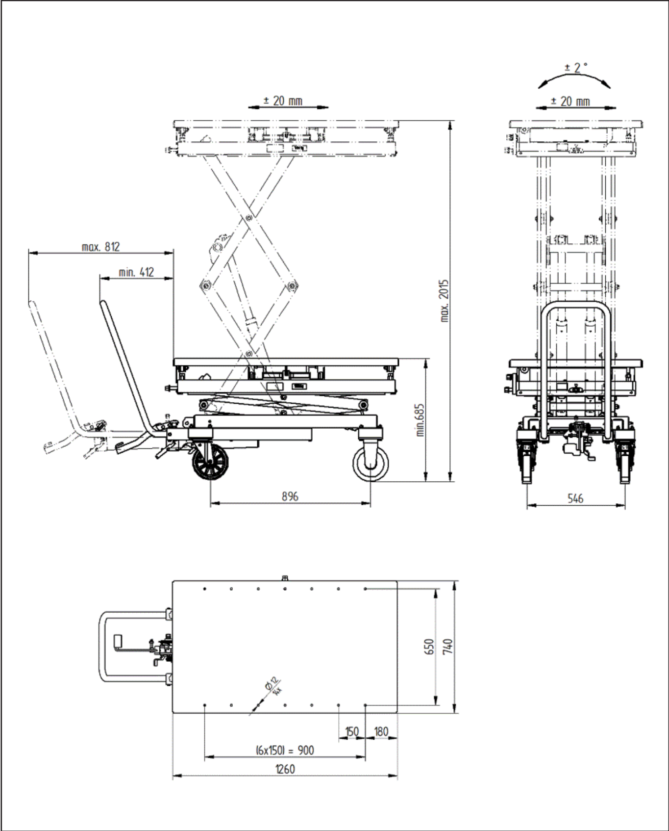
Hoja de medidas Master Gear S3 1.0 con extraíble
