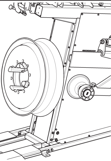
Blocage sur le trou central
