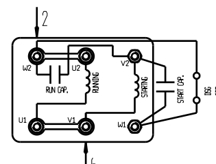
PODŁĄCZENIE SILNIKA ICME
