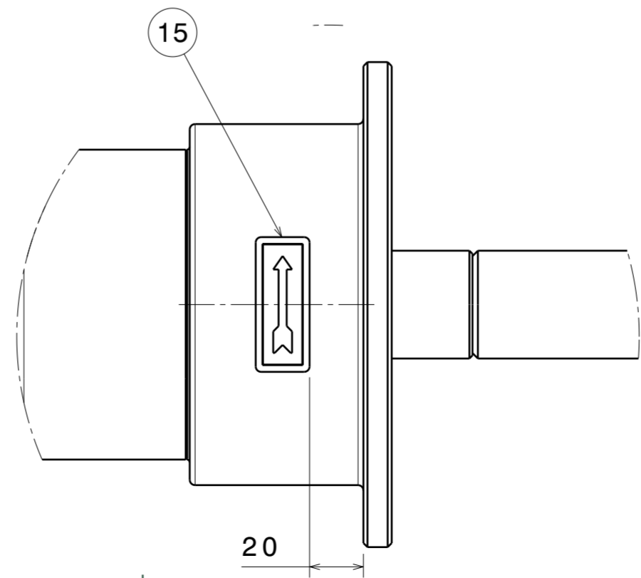
Dettaglio E Scala: 1:2
