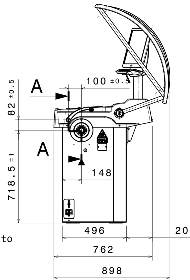
Vista Destra Scala: 1:15
