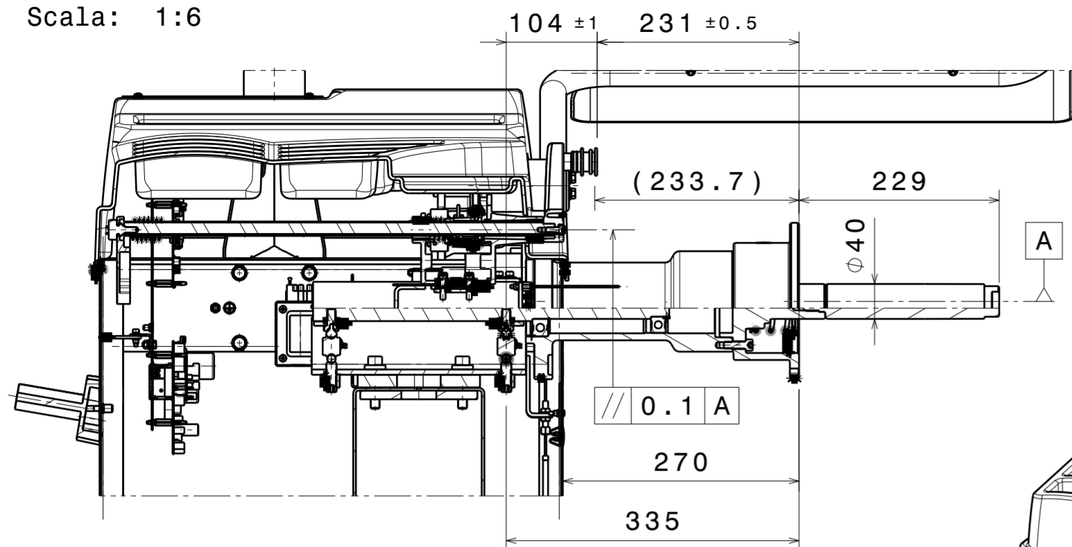
Vista in sezione A-A Scala: 1:6
