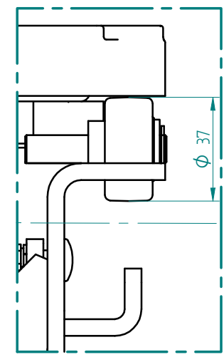
DETTAGLIO A
